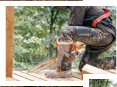
Sind alle Bodenbalken verlegt, wird der Rand mit der Säge „glattgezogen“.
