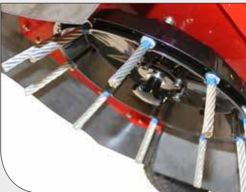
Werkzeuggesteller mit Schnellwechselsystem zum Borstenwechsel.
