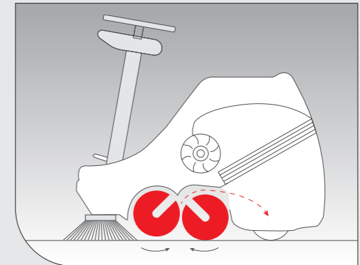
Die gegenläufigen Kehrwalzen des Doppelwalzensystems befördern Kehrgut in den Behälter.
