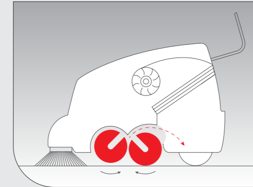
Durch das Doppelwalzensystem wird das Kehrgut mit Hilfe der gegenläufig rotierenden Kehrwalzen aufgenommen und in den Behälter befördert.
